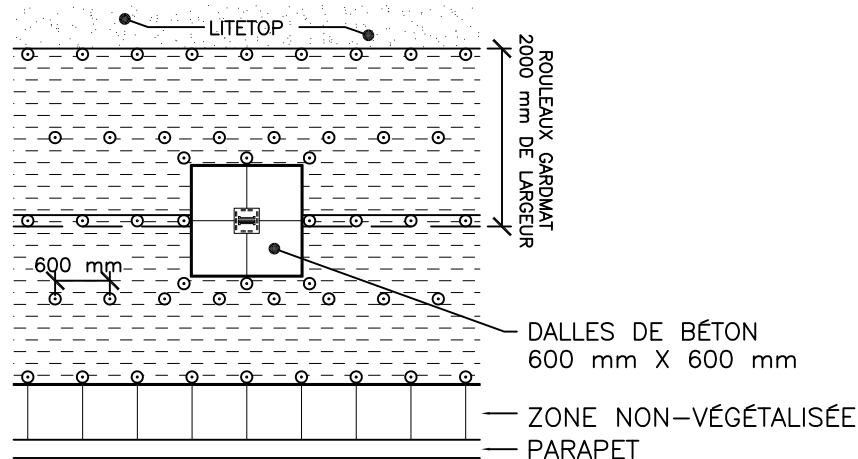
PETITE PÉNÉTRATION (i.e. DRAIN DE TOIT-COL DE CYGNE)
