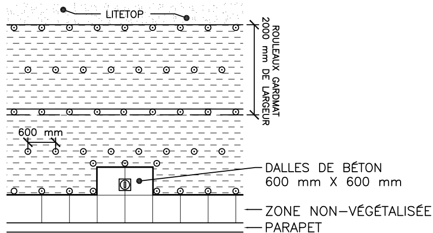
PÉNÉTRATION AU PÉRIMÈTRE (i.e. ANCRAGE POUR ÉCHAFAUDAGE)
