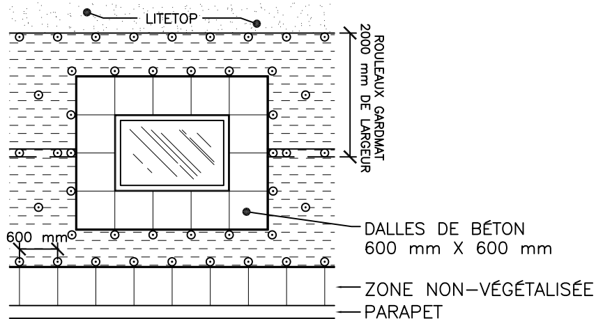
LARGE PÉNÉTRATION (e.i. Puits de lumière-suppport pour air climatisé)
